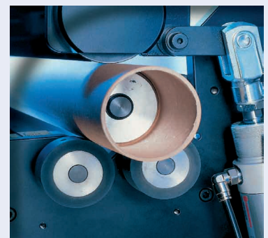
Coupeuse rotative.
